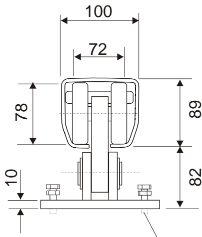
Höhenverstelle schraube
