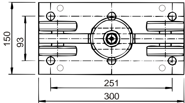
Bodenplatte Rollenbock
