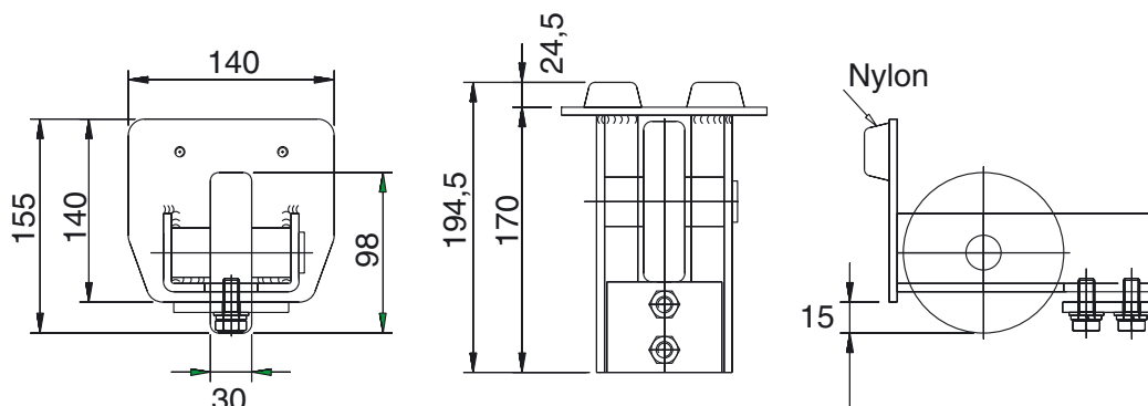
Rollenendstück
